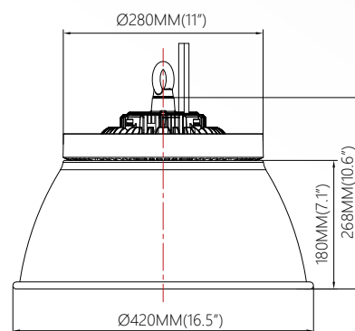
Reflector(Options)
